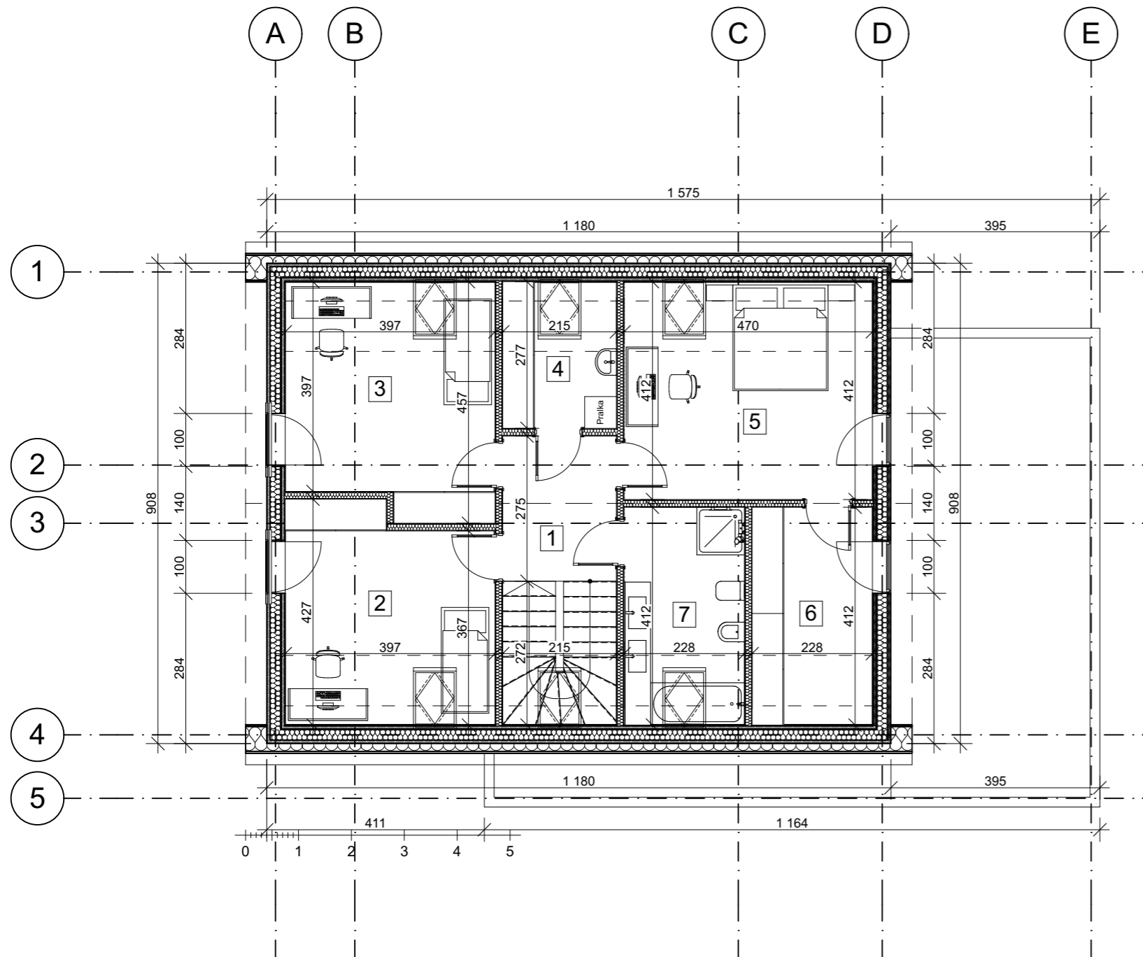
Poziom +1
